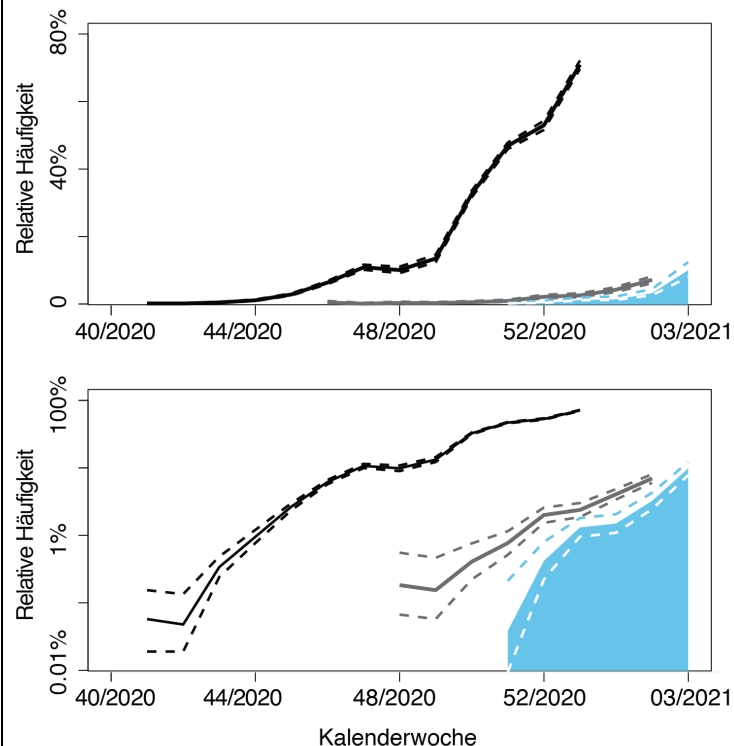
Abbildung 1: Entwicklung der relativen Häufigkeit (als Prozentsatz) aller positiven Tests, die auf B.1.1.7 zurückzuführen sind, in Grossbritannien (schwarz), Dänemark (grau) und der Schweiz (blau). Dieselben Daten sind auf einer linearen Skala (oben) und einer logarithmischen Skala (unten) dargestellt. Die untere Darstellung zeigt, dass der Anstieg in den drei Ländern anfänglich ungefähr exponentiell mit einer ähnlichen Geschwindigkeit erfolgt.
