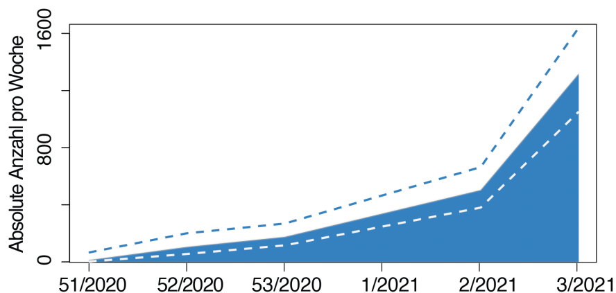
Abbildung 3: Schätzung der absoluten Anzahl der Infektionen mit B.1.1.7 pro Woche in der Schweiz. Zu beachten ist, dass die horizontale und die vertikale Achse anderes skaliert ist als in Abbildung 2.
