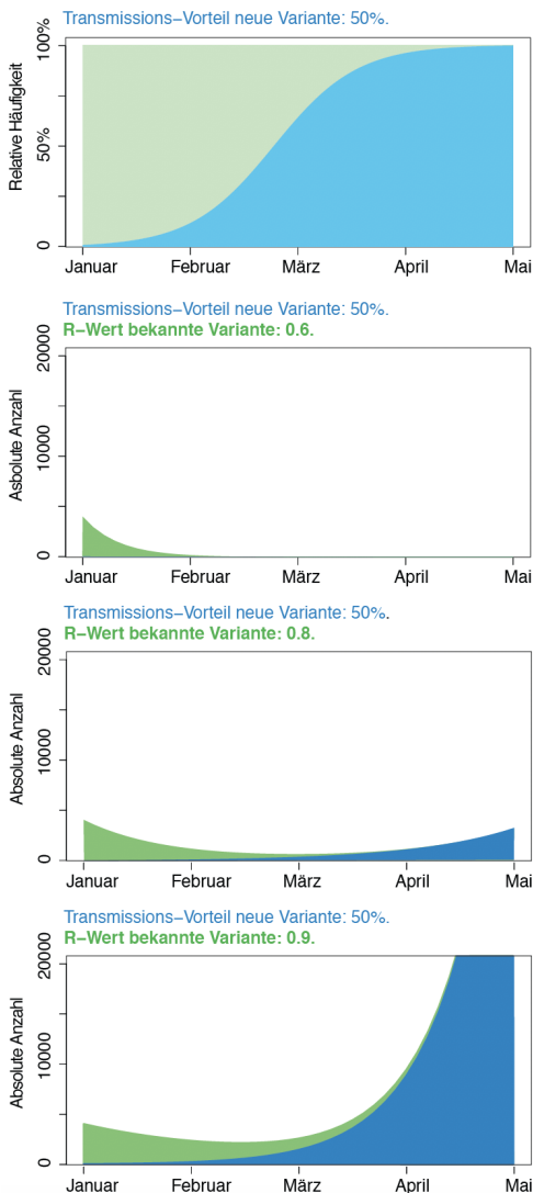
Abbildung 2: Einfaches numerisches Beispiel zur Illustration der Änderung der relativen Häufigkeit und der absoluten Anzahl einer Variante mit erhöhter Transmission. In allen vier Panels werden zwei Varianten dargestellt, eine alte Variante (grün) und eine neue Variante (blau) mit einer 50% höheren Transmissionsrate. A) Änderung der relativen Häufigkeit der neuen Variante (in blau) über die Zeit. Die Änderung in der relativen Häufigkeit verläuft für alle untenstehenden Szenarien gleich, unabhängig davon, ob die Fallzahlen insgesamt steigen oder fallen. B) Absolute Anzahl der Infektionen mit beiden Varianten pro Tag (alte Variante in grün, neue Variante in blau) in einer Situation, in der der R-Wert für die alte Variante 0.6 beträgt. Dies ist eine Situation, in der wirkungsvolle Massnahmen und eine gute Umsetzung die Ansteckungen rasch reduzieren können. C) Absolute Anzahl der Infektionen mit beiden Varianten pro Tag (alte Variante in grün, neue Variante in blau) in einer Situation, in der der R-Wert für die alte Variante 0.8 beträgt. D) Absolute Anzahl der Infektionen mit beiden Varianten pro Tag (alte Variante in grün, neue Variante in blau) in einer Situation, in der der R-Wert für die alte Variante 0.9 beträgt. Dieses Beispiel macht eine Reihe von vereinfachenden Annahmen. Es dient deshalb nur der Illustration der Überlegungen im Haupttext, und soll nicht als Prognose der tatsächlichen Entwicklung der Infektionen in der Schweiz interpretiert werden. Insbesondere berücksichtigt dieses Beispiel Immunisierung durch Impfung oder kürzlich durchgemachter Infektion nicht. Mehr Details zu diesem Beispiel finden sich im wissenschaftlichen Update vom 29.12.2020 16 .
